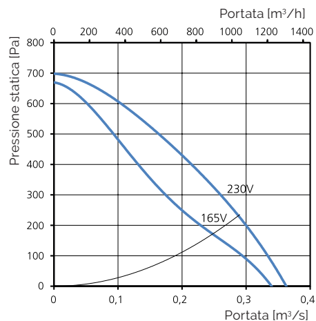
RKB 500x250 E1
