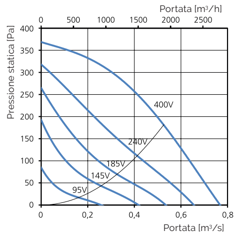
RKB 600x350 B3
