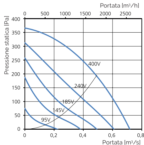
RKB 600x300 B3
