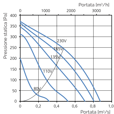
RKB 600x300 C1
